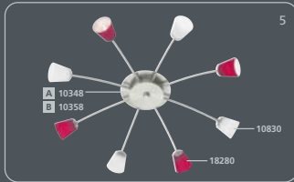
Ø 52 cm incl. Ooram G9 / 25 W
