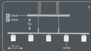
incl. G4 12 V / 20 W
